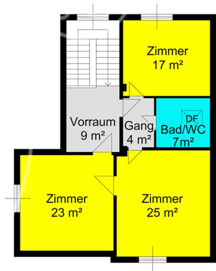
DF ... Dachfenster Skizze Dachgeschoss
