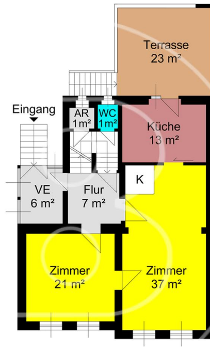
VE ... Veranda K ... Kaminofen AR ... Abstellraum Skizze Hochparterre
